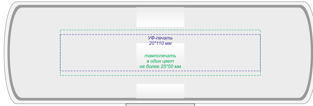
футляр вид сверху
